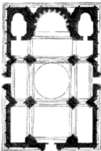
Č. 272. Kathedrála v Ani (půdorys).
