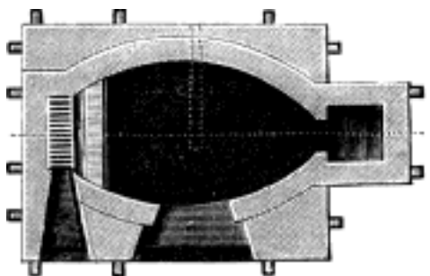
Č. 293. Pec plamenná (průřez horizontální).
