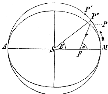
Č. 276. Anomalie (astron.).
