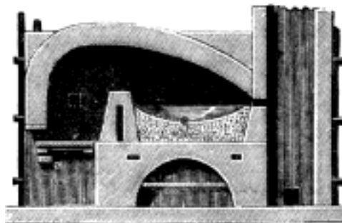
Č. 292. Pec plamenná (průřez vertikální).
