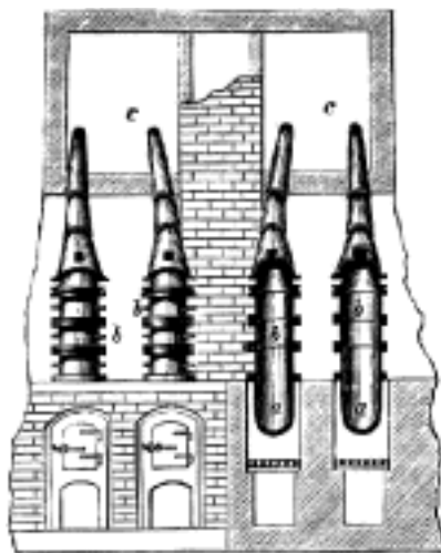
Č. 349. Apparát sublimační.
