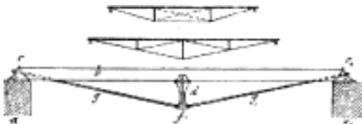
Č. 342. Armatura trámová.
