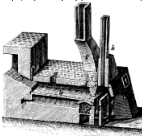
Č. 348. Pec muflová v Reichensteině.
