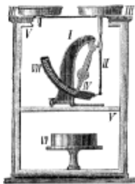
Č. 377. Atmometr Wildův.
