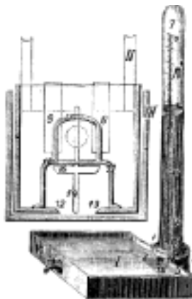
Č. 376. Atmometr Prestelův.
