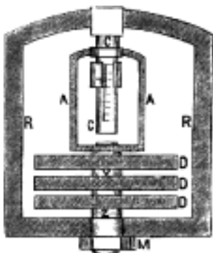
Č. 478. Bathometr Hopfgartnerův.
