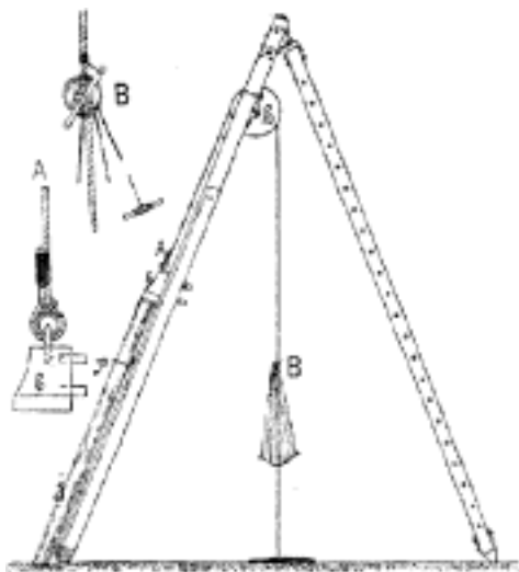
Č. 530. Beranidlo tahací.
