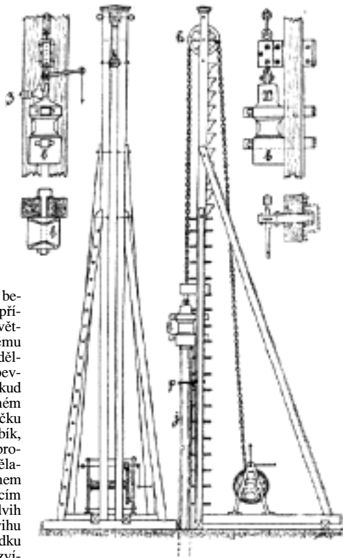
Č. 531. Beranidlo strojové.
