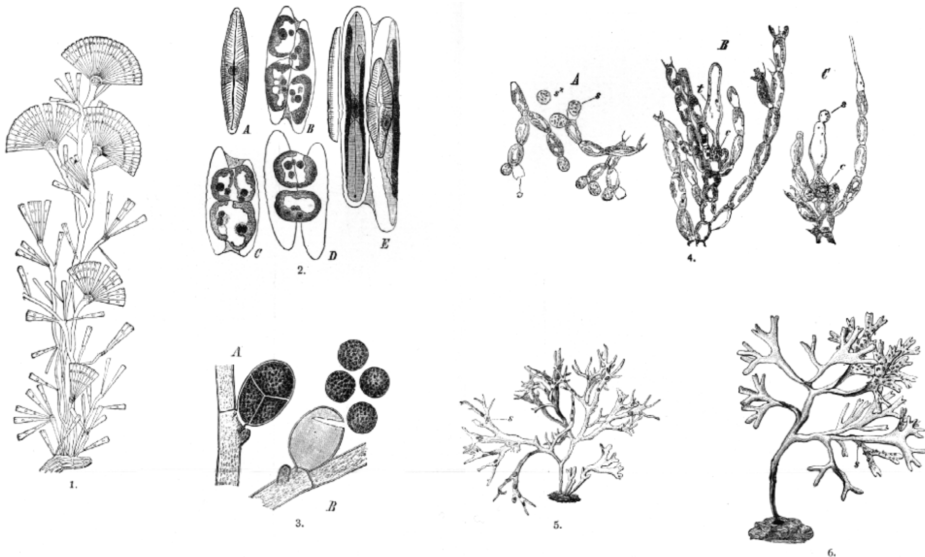
Obr. 1. a 2. Rozsivky. - Obr. 3. - 6. Řasy ruduchovité.
