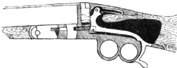
18. Lůžkový závěr s klínkem a dlouhou pakou (vzor »Ideal«).
