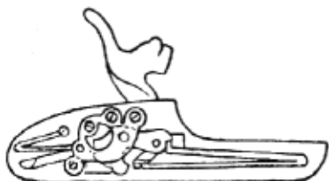
1. Ručníční zámek stranní (vnitřní zařízení).
