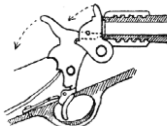
7. Závěr a zámek Remingtonův, zavřený.
