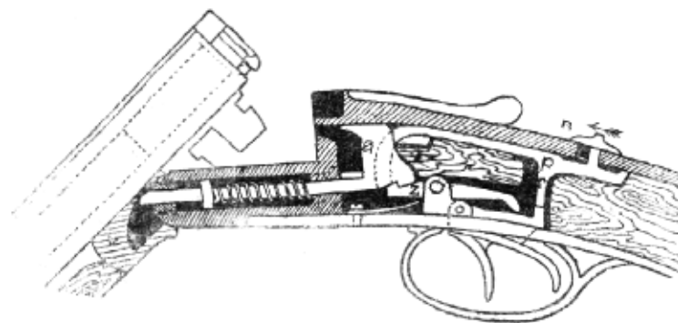
17. Ručnice bez kohoutků (vzor Schlegelmilchův) se spirálními zátky; natahují se samočinně při sklonění hlavní.
