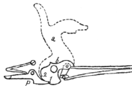
3. Ručníční zámek s odskakujícím kohoutkem. a kohoutek, b ořech, p západka. Při spuštění zámku stavi se kratší rameno zpruhy pod rameno ořechu, následkem čehož se kohoutek po úderu zvedne do výše prvního západu.
