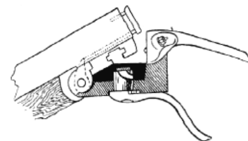
12. Lůžkový závěr s klíčem k zadu položeným.
