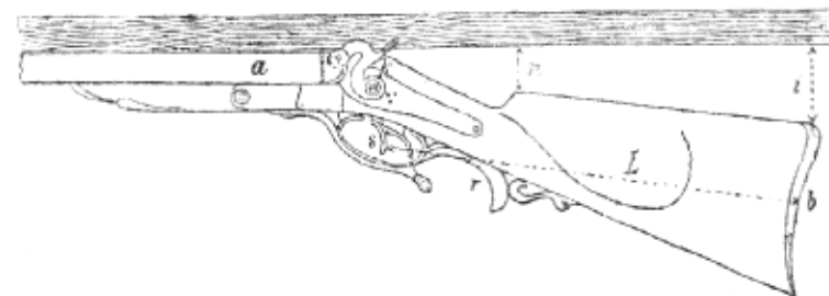
19. Měření pažby: a hlaveň, b botka, L lícnice, s - b délka pažby od spouště k bodce; n křivost nad nosem pažby, i křivost pažby nad botkou.
