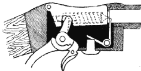
10. Závěr sklonným špalíčkem podle Peabodyho, zavřený. V závěrním špalíčku jest umístěn válcovitý (spirální) zámek.
