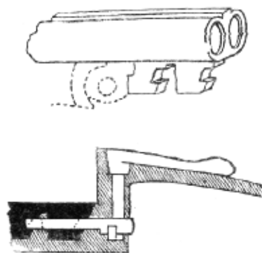
14. Lůžkový závěr s klínkem dvojnásobně zapadajícím a pakou nahoře umístěnou. - Hlavně k závěru tomu náležející.
