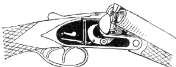
16. Ručnice bez kohoutků; zámky natahují se samočinně při sklonění hlavní.
