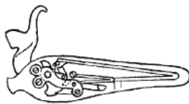
2. Ručníční zámek zpětný (vnitřní zařízení).
