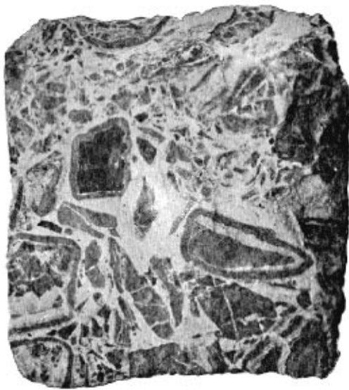
Brekcie žilná, tak nazv. »ruda kroužková« z Zellerfeldu na Harcu. Ostrohrané úlomky pískovce a břidlice jsou obaleny galenitem, sfaleritem a křemenem. Dle R. Becka.
