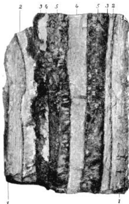
Souměrná výplň žíly v Příbramě (Ševčínská žíla, 22. obzor). 1. droba, 2. siderit, 3. sfalerit, 4. kalcit, 5. galenit. Fotogr. prof. Ad. Hofmann v Příbrami.
