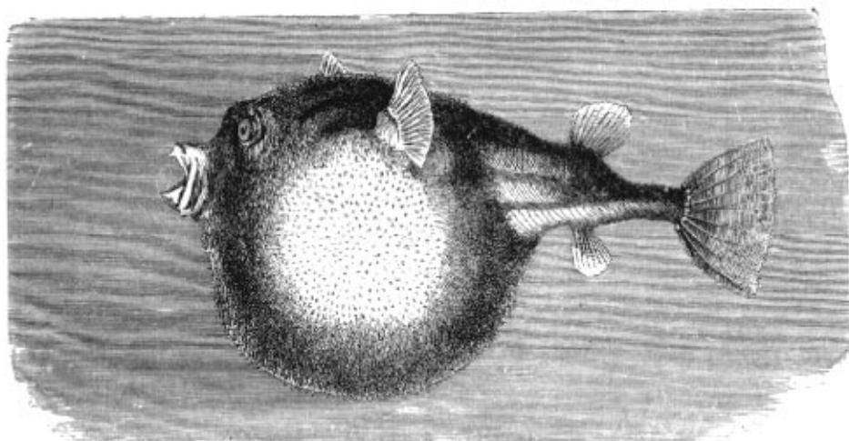
Nahozubci (ryby srostločelistné): Čtverozubec pruhovaný ( Tetrodon fahaka ).
