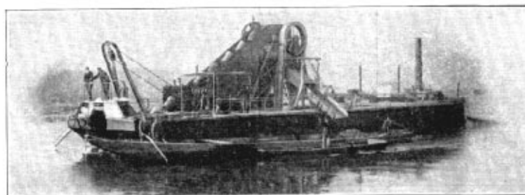
Rýpadlo mnohoputné při práci u Troje na Vltavě r. 1889.
