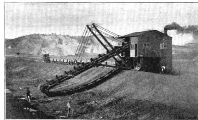
Rýpadlo mnohoputné při stavbě přístavu holešovického.
