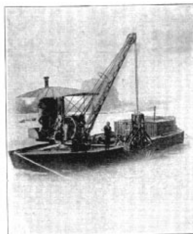
Drapák Priestmanův při práci u Troje na Vltavě r. 1889.
