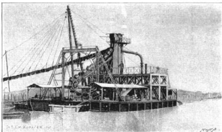
Rýpadlo ku skládání splachováním. (Elevator.)
