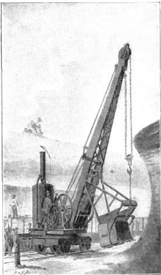
Rýpadlo rýčové Whitakerovo.
