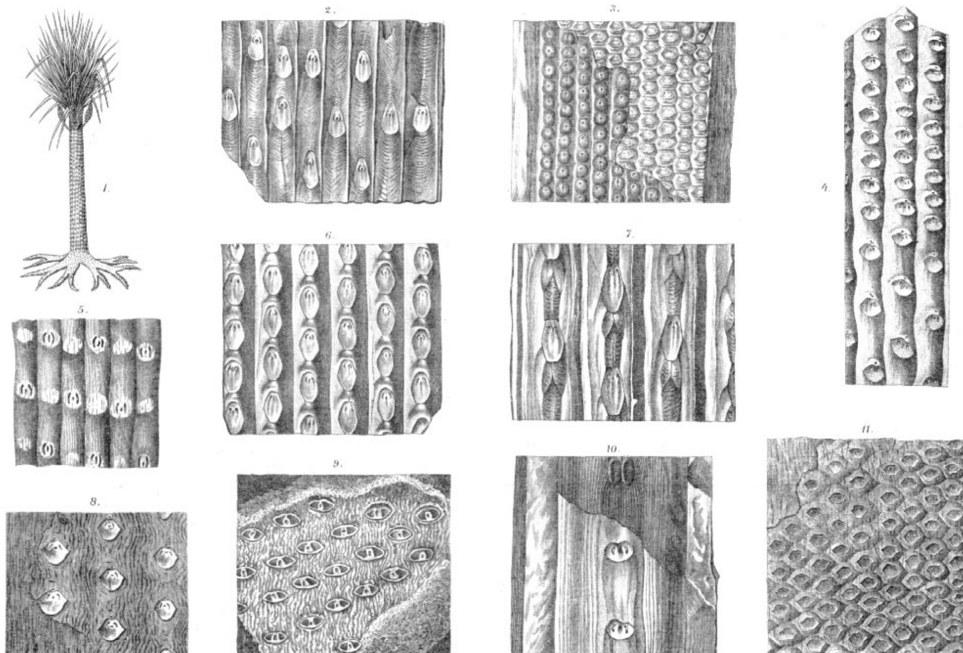
1. Restaurovaný strom sigillarie ( Eusigillaria ) s kmenem v dol. 2/3 jízvami po odpadlých listech posetým a dole v kořenovité oddenky ( Stigmara ) se rozvětvojícím. 2. S. Sillimani Brongn. 3. S. elegans Brongn. 4. S. s dvojitou skulpturou: nahoře tessellantní, dole rhytidolepickou. 5. Dekortikát Sigillarie . 6. S. elliptica Brongn. 7. S. elongata Brongn. 8. S. Brardi Brongn (f. denudata ). 9. S. oculina Blankenh. 10. S. reniformis Brongn. 11. S. Brardi Brongn s dvojitou skulpturou.
