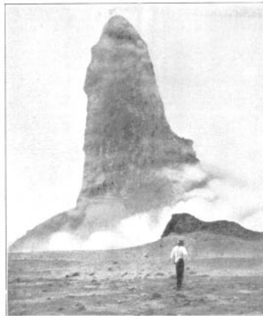
Jehlan lávový 350 m vysoký, vzniklý za výbuchu sopky Mont Pelée v jejím jícnu. Podle E. O. Hoveye.
