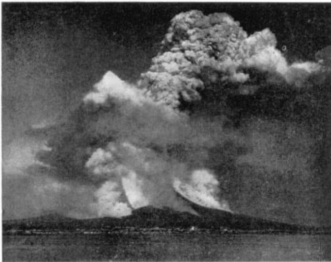
Výbuch sopky Vesuvu r. 1872.
