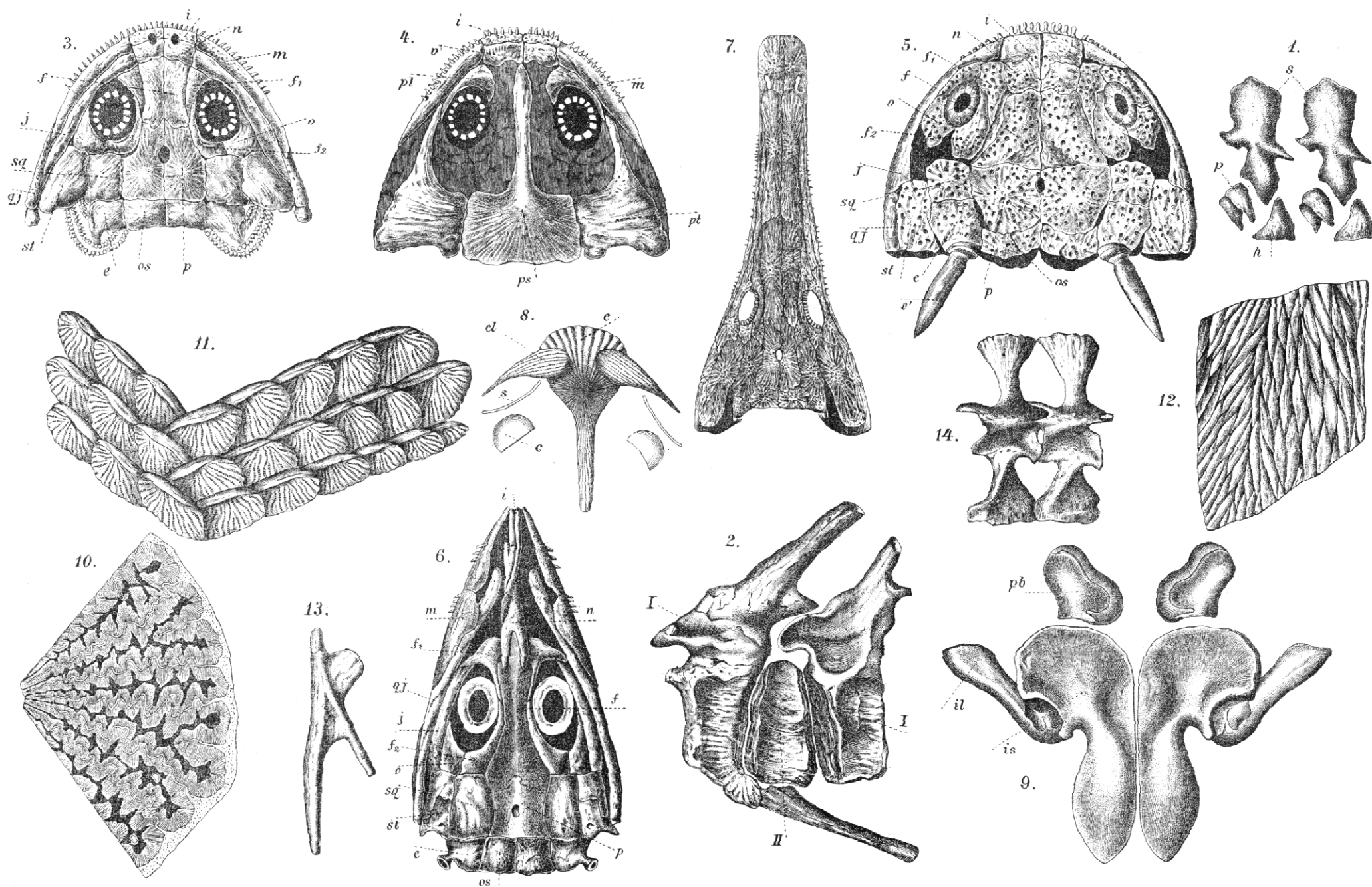
1. Rhachitomní obratle ocasní r. Archegosaurus, s svrchní oblouky, p pleurocentrum. - 2. Embolométní obratel r. Diplovertebron, I. svrchní oblouk s hypocentrem, II. pleurocentrum. - 3. Branchiosaurus salamandroides lebka shora, i mezičelist, m čelist, n nosní, f1 přední, f2 zadní, f čelní kost, p temenní, o zaočnicová, sq skořepová, j jářmová, qj čtverečnojářmová, st svrchní skráňová, e přední sluchová, os svrchní týlní. - 4. Týž druh, lebka zdola ps parasfenoid, pt křídlová, pl podnebí, v rádlová, m čelist, i mezičelist. - 5. Keraterpeton crassum lebka shora, vysvětlivky jako u čís. 3. - 6. Dolichosoma longissimum lebka shora, vysvětlivky jako u čís. 3. - 7. Archegosaurus Decheni lebka s hory. - 8. Melanerpeton, pás plecový, e episternum, cl clavicula, s scapula (sleithrum), c coracoid (scapula). - 9. Mastodonsaurus, pás bederní, il kyčelní, is sedací, pb stydká. - 10. Příčný řez zubem r. Mastodonsaurus. - 11. Část břišního pancíře dr. Limnerpeton obtusatum. - 12. Část břišního pancíře dr. Ophiderpeton vicinum. - 13. Žebro dr. Ophiderpeton granulosum. - 14. Dva ocasní obratle dr. Urocordylus scalaris.
