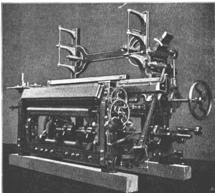
Strojní stav na damašky (soustava Oberleithnerovy).
