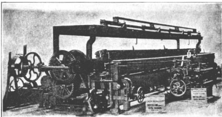
Strojní stav na plachty a úzký stav anglický (na bavlnu).
