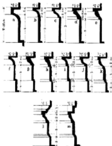
Č. 1890. Profily chambrany.
