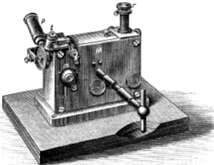
Č. 1931. Siemensův chronograf.
