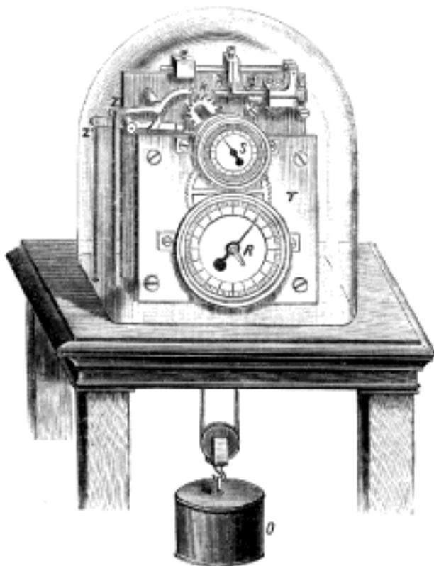
Č. 1933. Hippův chronoskop.
