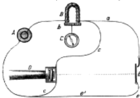
Č. 1932. Wheatstoneův chronoskop.
