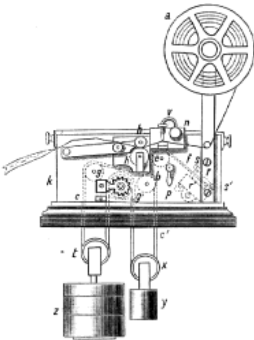
Č. 1929. Hippův proužkový chronograf.
