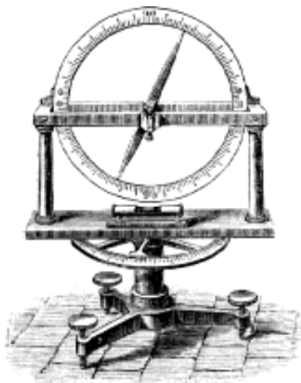
Č. 1971. Inklinatorium.
