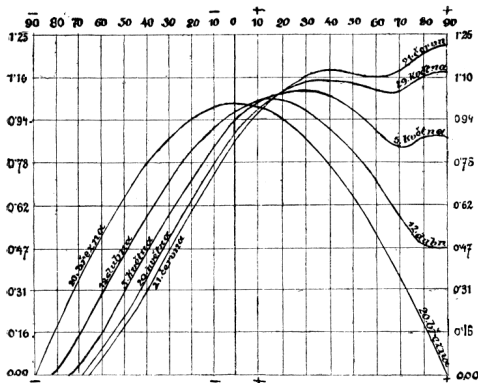
Č. 1973. Rozdělení slunečního ozáření na povrchu zemském v době od jarní rovnodennosti do letního slunovratu, bez ohledu na atmosférickou absorpci.
