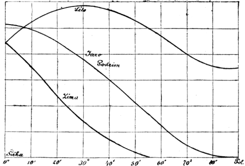
Č. 1974. Velikost insolace dle zeměpisné šířky a dle ročních dob.
