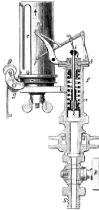
Č. 1955. Indikátor soustavy Rosenkranzovy .
