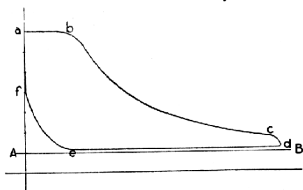
Č. 1957. Indikátorový diagram.
