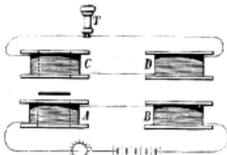
Č. 1965. Indukční váha.
