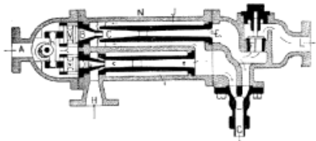
Č. 1969. Universální injektor Körtingův.
