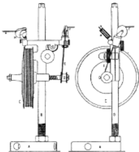
Č. 1956. Staňkův reduktor zdvihu.
