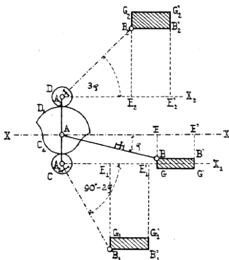
Č. 1978. Theoriae integratorum.
