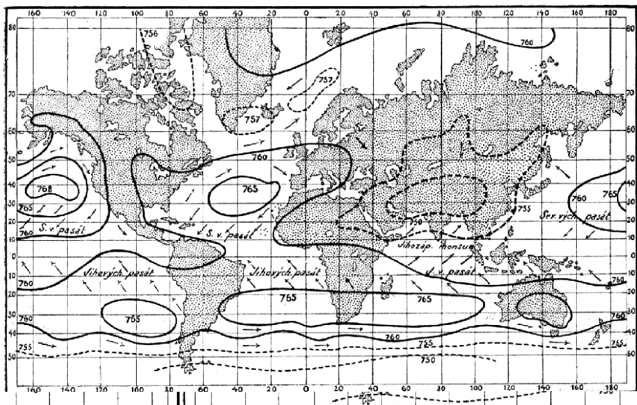
Č. 1992. Isobary v červenci. Vysoký tlak. Nízký tlak. Šípky označují panující směr větru.
