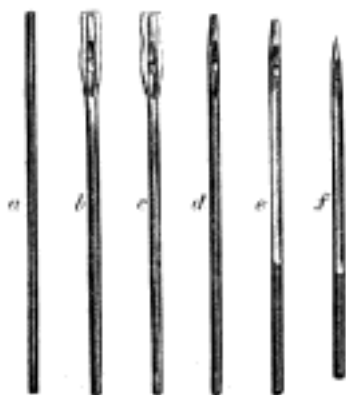
Č. 2027. Jehlářství (výroba jehel strojových).
