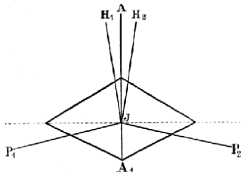
Č. 2033. Jelletovo prisma.
