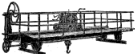
Č. 2051. Jeřáb posuvný.
