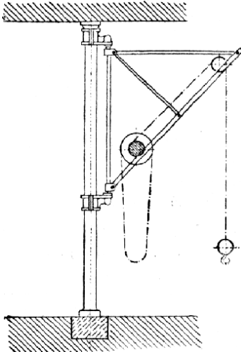
Č. 2038. Jeřáb skladištní na sloupu.
