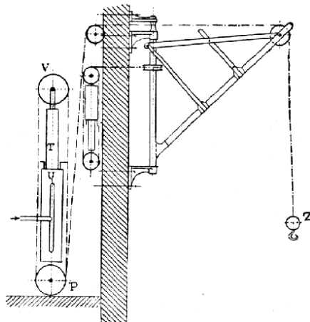
Č. 2042. Schéma jeřábu nástěnného s hydraulickým pohonem.
