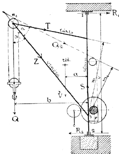
Č. 2036. Schéma jeřábu skladištního.
