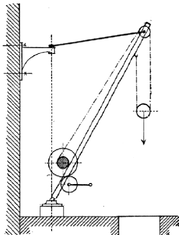
Č. 2037. Jeřáb otáčivý beze sloupu.
