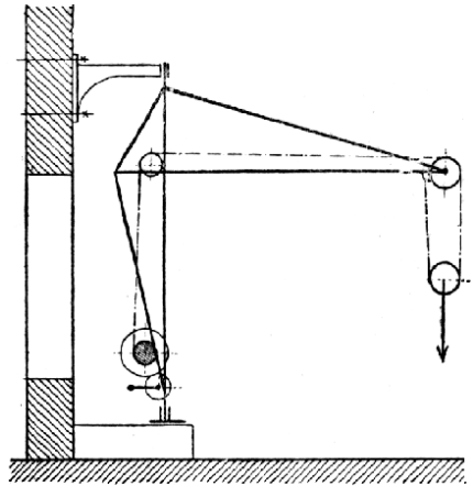
Č. 2040. Jeřáb skladištní beze vzpěry.
