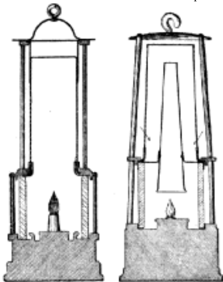
Č. 2118. Kahau Clannyův. Č. 2119. Kahau Müselerův.
