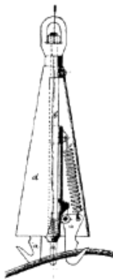
Č. 2113. Kabelová sonda.
