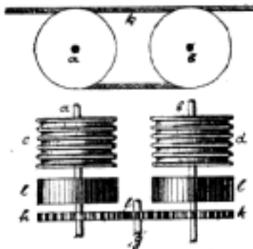
Č. 2112. Kabelová brzda.
