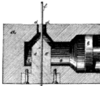
Č. 2104. Siemensův lis.
