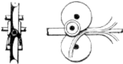
Č. 2103. Stroj na izolování drátů.
