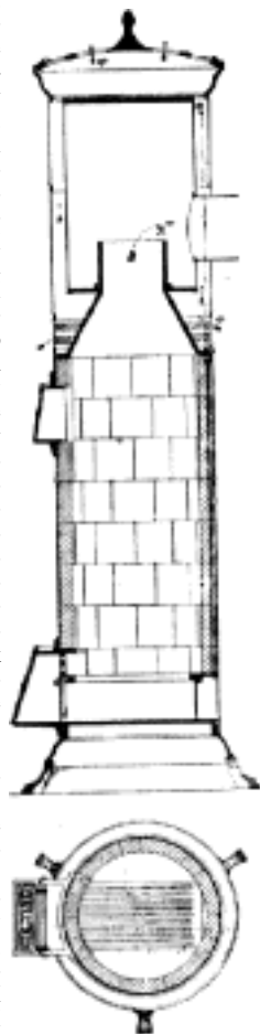
Č. 2146. Kamna plechová s vyšamotovaným ohništěm.
