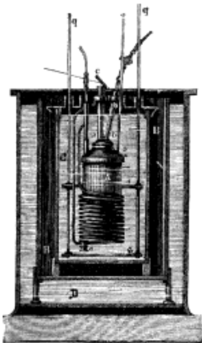
Č. 2132. Kalorimetr Favre-Silbermannův.
