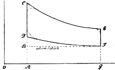
Č. 2126. Diagram kalorického stroje uzavřeného.
