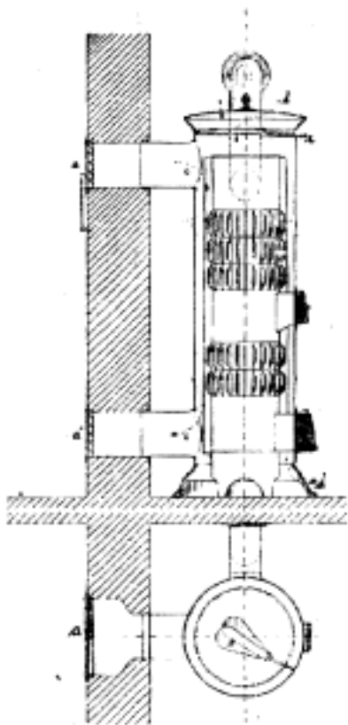
Č. 2149. Kamna Meidingerova k vytápění několika místnosti.
