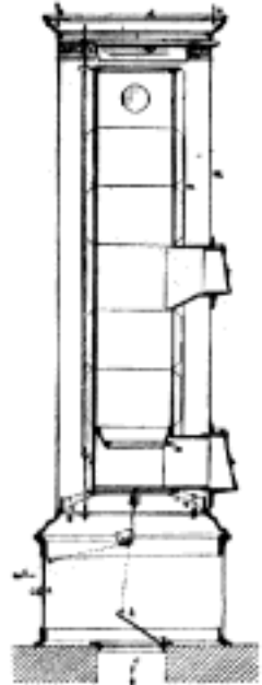
Č. 2148. Kamna Meidingerova s ventilačním topením a s miskou na odpařování vody.
