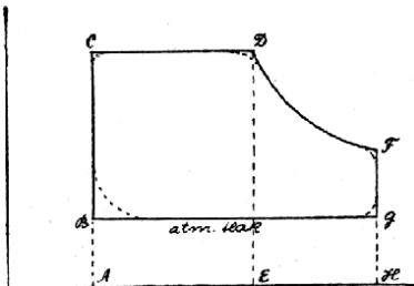
Č. 2123. Diagram kalorického stroje otevřeného.
