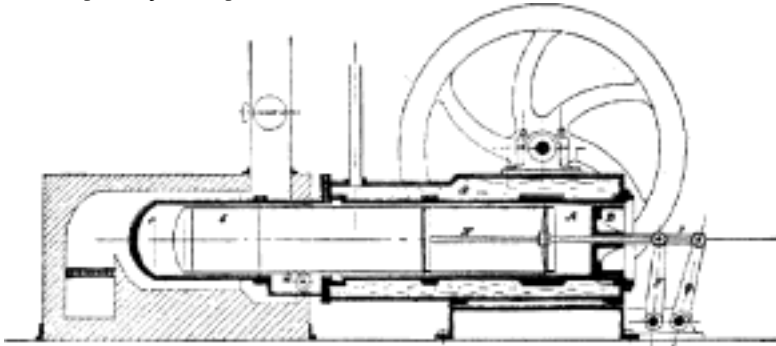
Č. 2127. Lehmannův kalorický stroj.
