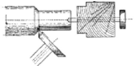
Č. 2143. Soustruhování tvrdých kamenů.
