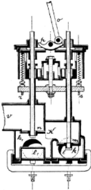
Č. 2125. Rozvod Hockova kalorického stroje.
