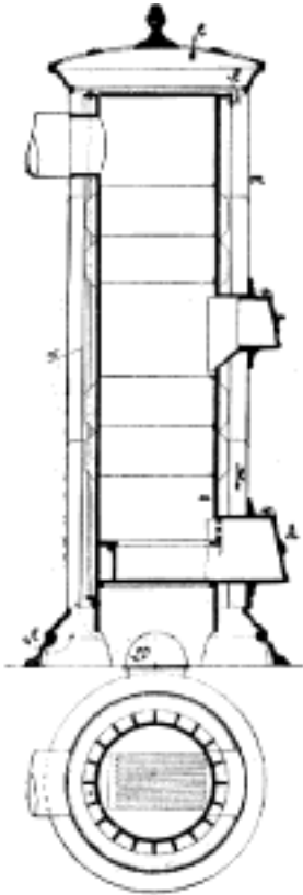
Č. 2147. Kamna Meidingerova.
