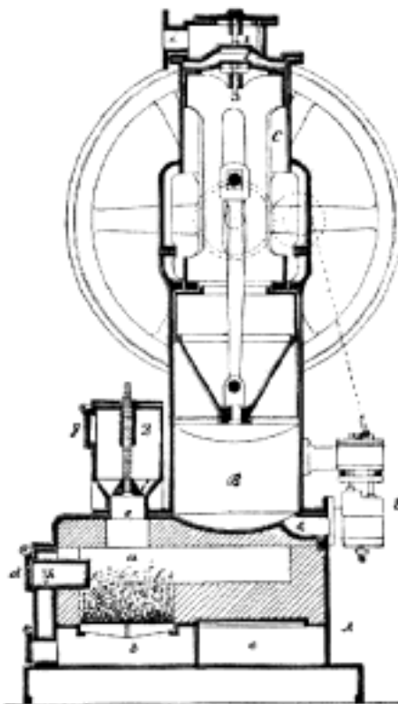
Č. 2124. Horký kalorický stroj.
