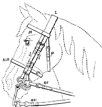
Č. 2156. Kantár občanský jezdecký, tak zv. anglický. z záhlavníku, n náčelek, n nánosek, II licnice, p podhrdlek, os ořez stihlová, ou ořez udidlová.
