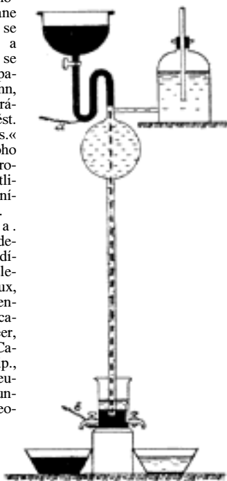
Č. 2163. Kapilární článek.
