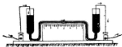
Č. 2164. Kapilární elektrometr.
