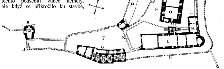
Č. 2169. Půdorys hradu Karlštejna z r. 1898. A Cesta v XVI. stol. as o 8 metrů snížená. B Voršílka, bývalá první brána, než byla cesta k ní vedoucí snížena. C Brána ze XVI. stol. D Cesta kolem hradb, ke druhé bráně vedoucí. E Brána druhá. F Náhradí před purkrabstvím. G Purkrabství. H Hradby dolejší se střilami. H1 Hradby hořejší se střilami. J Hlášky. K Brána k náhradí před císařským palácem. L Císařský palác. M Obydlí děkana kanovníků. N Náhradí druhé, povýšené. O Budova s kaplí P. Marie a sv. Kateřiny. P Náhradí nejvyšší. Q Budova s kaplí Sv. Kříže. R Věž, v níž jest studna. S Upatí Kněží hory.
