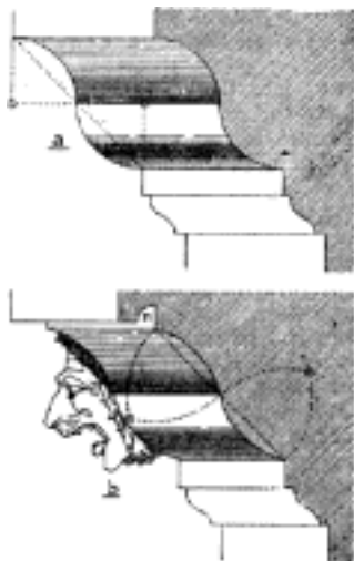
Č. 2170. Žlábkovnice č. sima.
