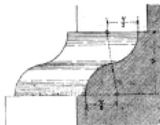
Č. 2173. Vzpěrnice č. obrácená laloška.
