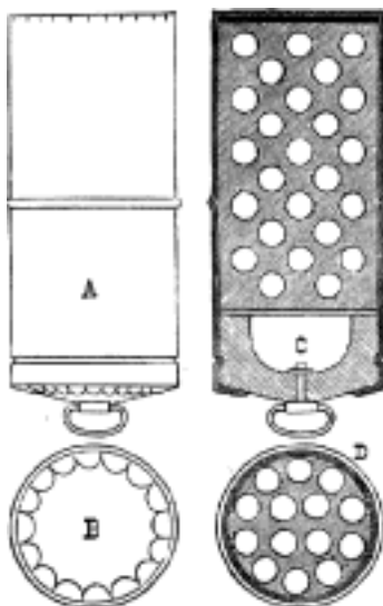
Č. 2174. Kartáč v dělostřelbě rakousko-uherské. A pohled vnější se strany, B pohled vnější shora, C průřez dle délky, D průřez příční.
