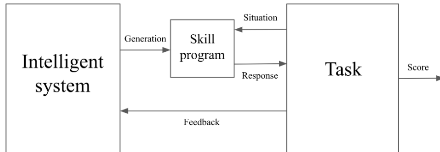
Figura 2.2: Posición del problema, un sistmema inteligente que genera programas de habilidades que interactúan con una tarea.
