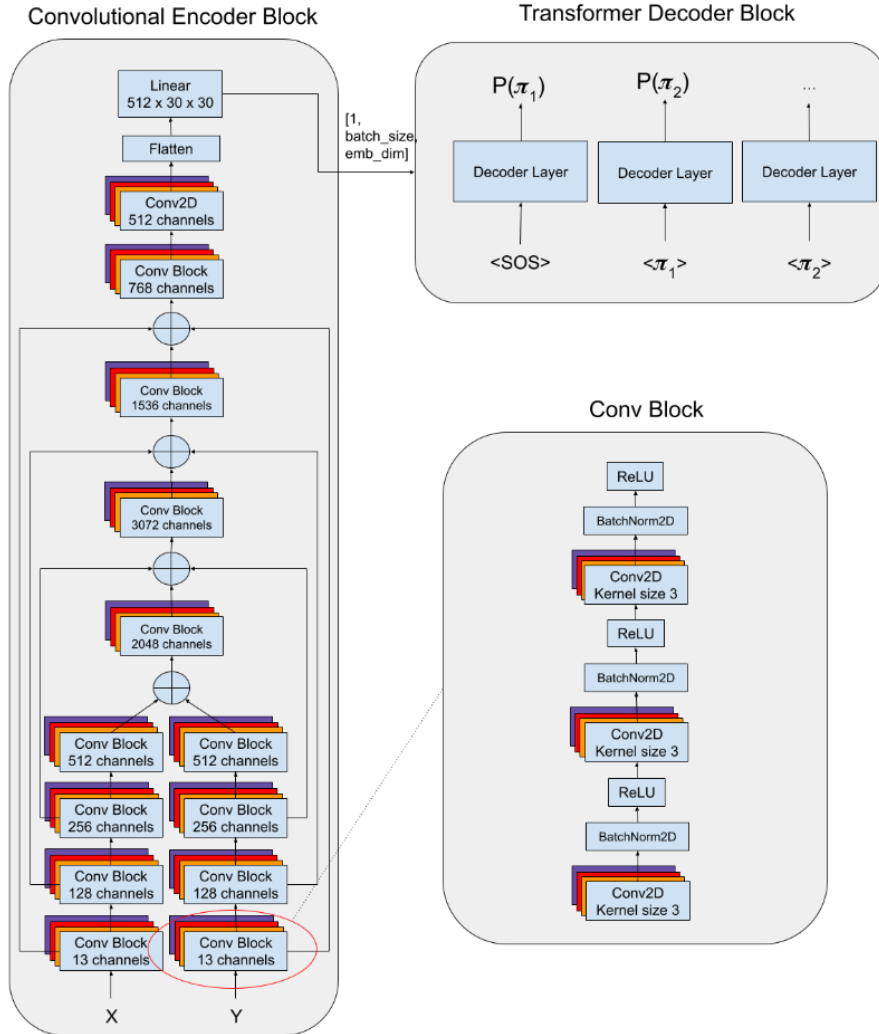
Figura 2.13: Arquitectura VLM utilizada en GridCoder.
