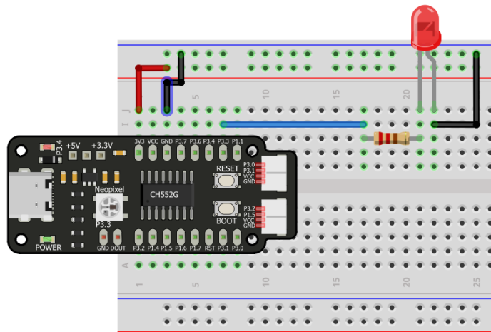
Figura 2.8: LEDs
