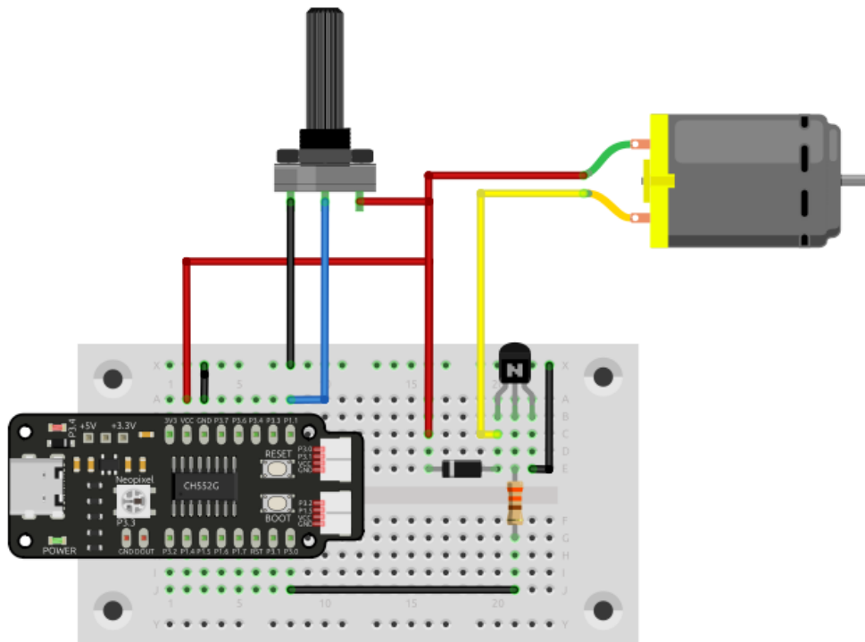
Figura 2.13: Control de velocidad de un motor por PWM con entrada analógica
