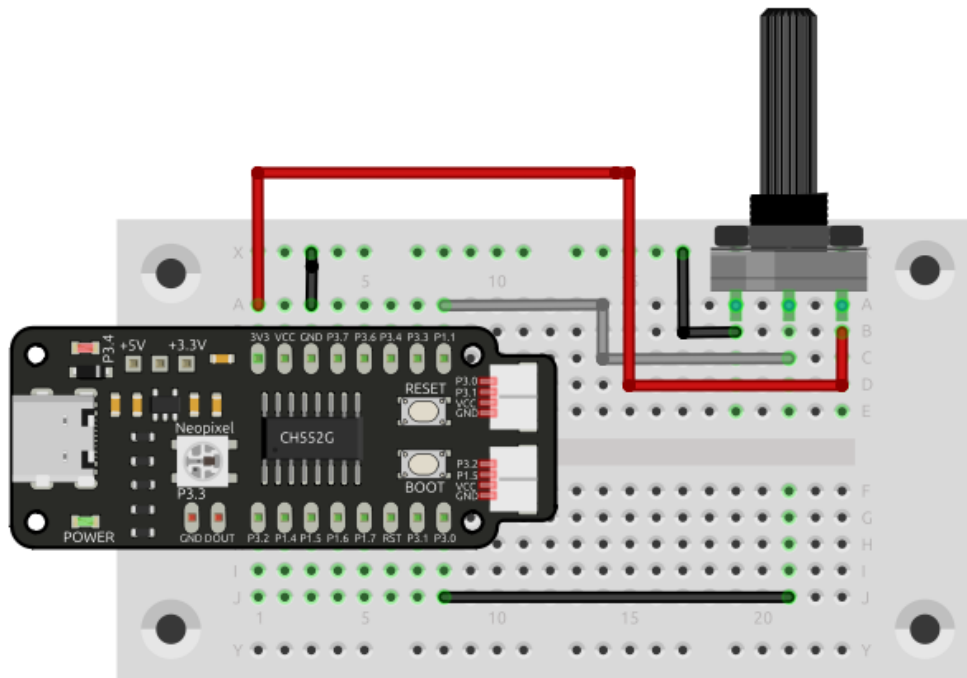
Figura 2.13: Lectura de potenciómetro salida serial
