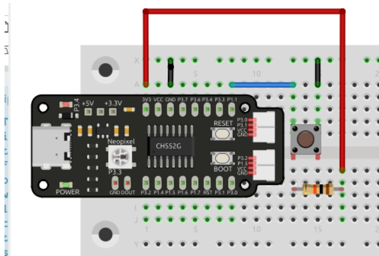
Figura 2.11: Aplicación de entrada digital
