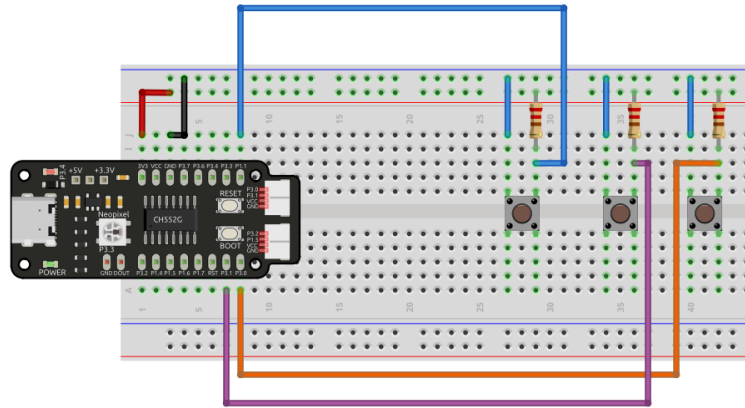
Figura 2.17: Ejemplo de Dispositivo HID
