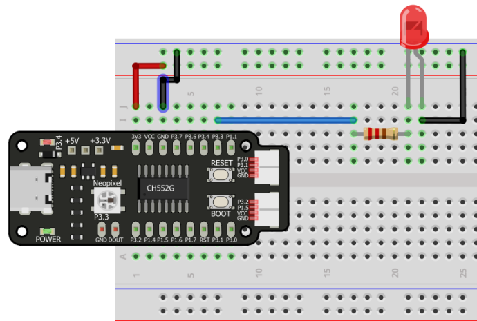
Figura 2.8: LEDs
