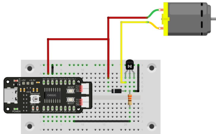
Figura 2.10: Controlador de velocidad de motor
