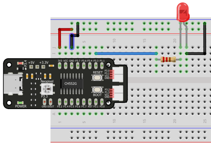
Figura 2.9: LEDs
