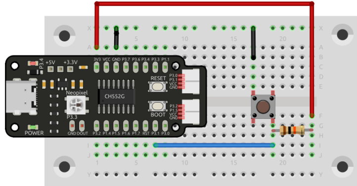
Figura 2.18: Aplicación de entrada digital
