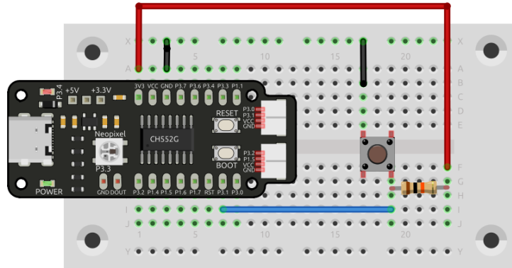
Figura 2.12: Aplicación de entrada digital
