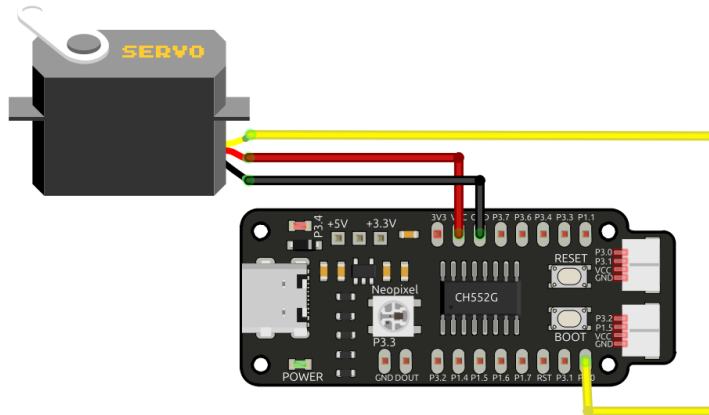
Figura 2.11: Controlador de servomotor
