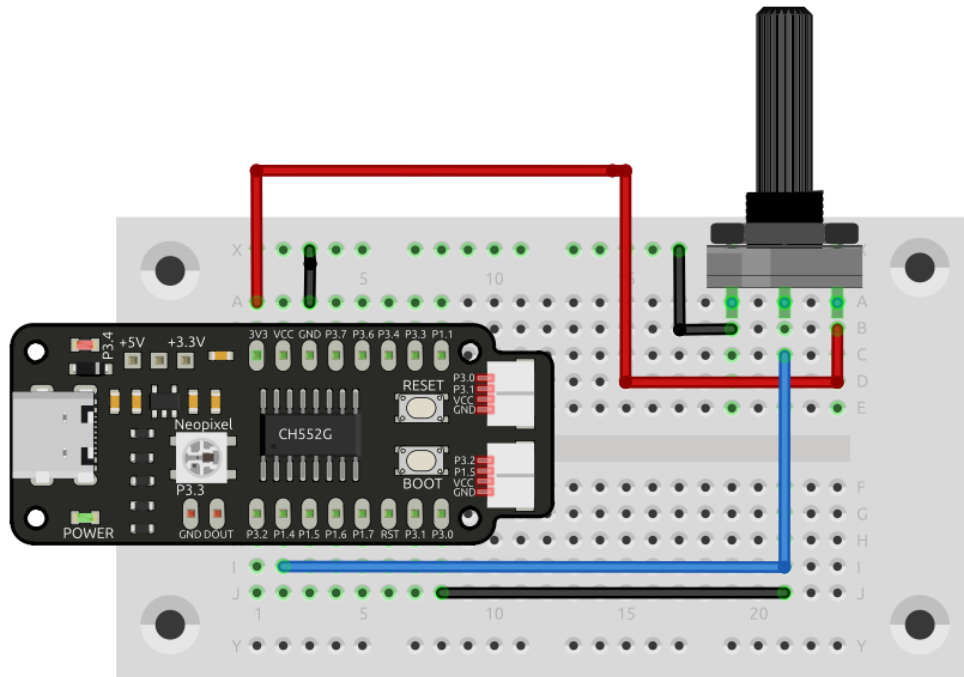
Figura 2.14: Lectura de potenciómetro salida serial
