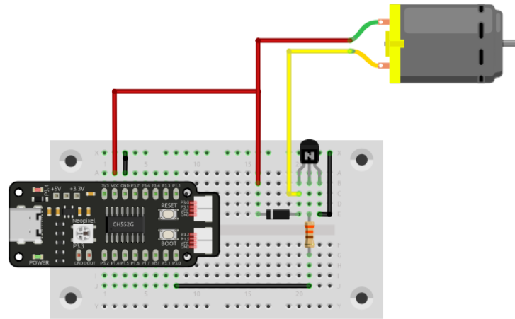
Figura 2.11: Controlador de velocidad de motor
