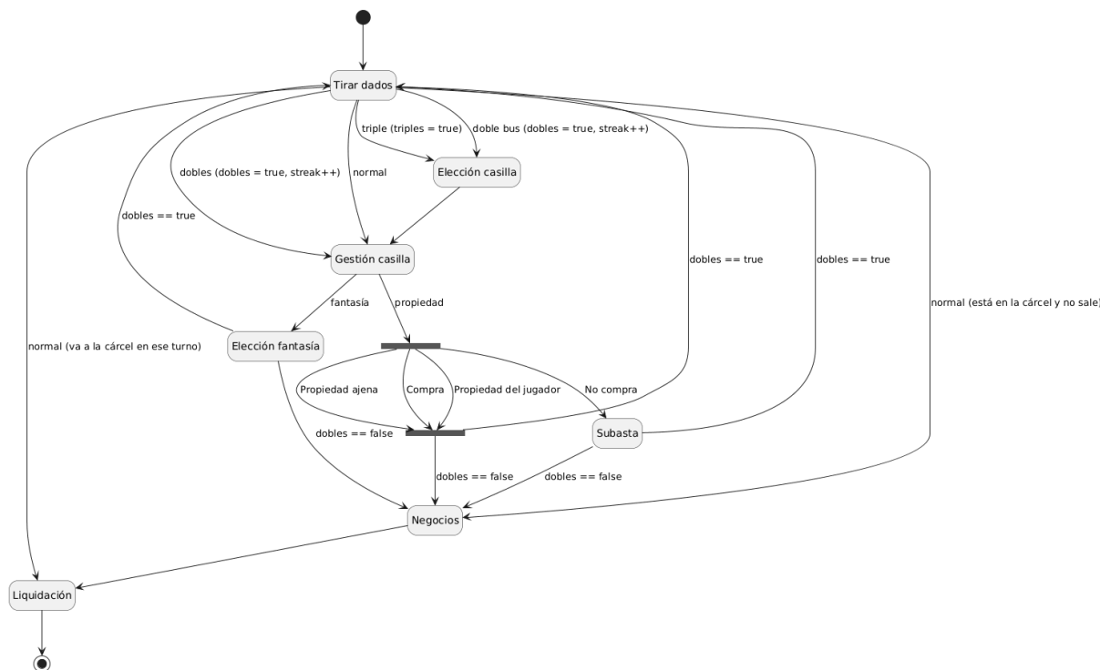
Figura 4: Diagrama de estados de un turno de juego con sus fases.
