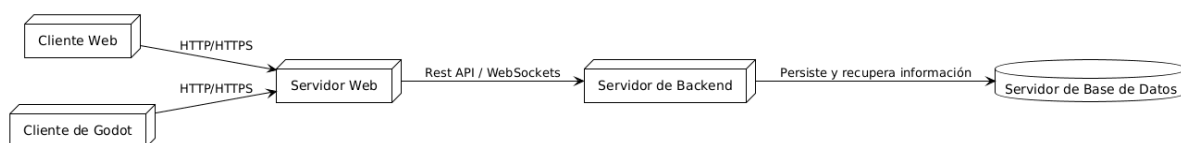
Figura 3: Diagrama de la arquitectura a alto nivel.
