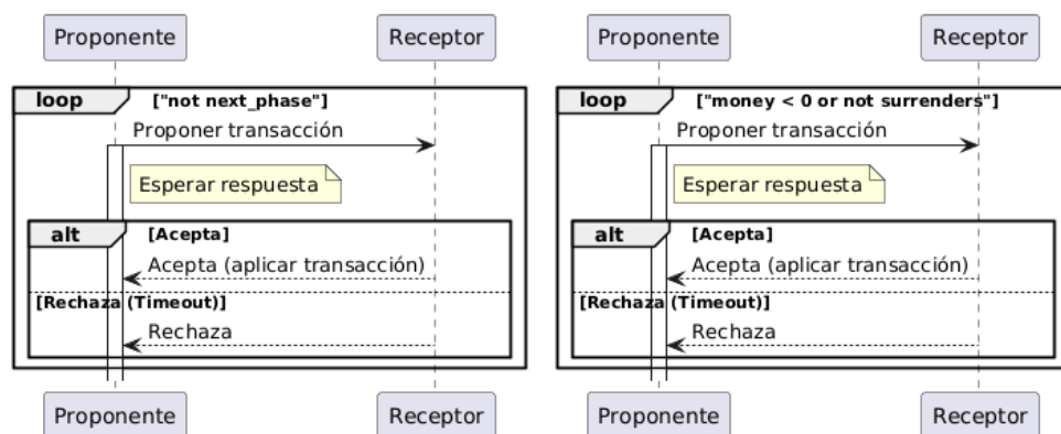
Figura 5: Diagramas de secuencia de las fases de negocios (izquierda) y liquidación (derecha).
