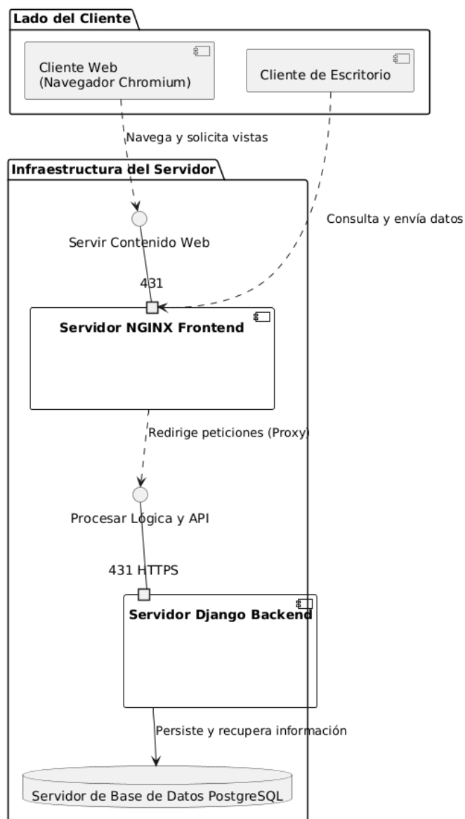
Figura 26: Diagrama de componentes y conectores.
