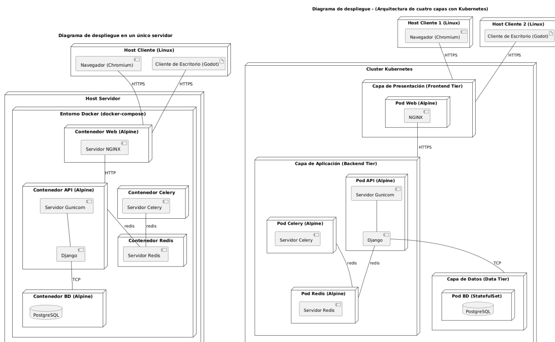
Figura 6: Diagramas de despliegue. A la izquierda, diagrama en 2 capas, como se realizará el despliegue, y a la derecha, en 4 capas, señalando las posibilidades de despliegue.
