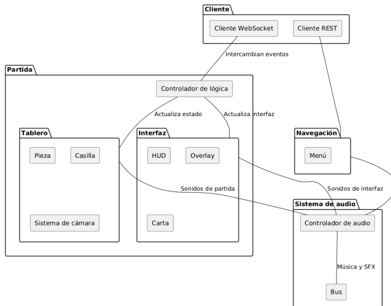
Figura 29: Diagrama de módulos del cliente de escritorio.
