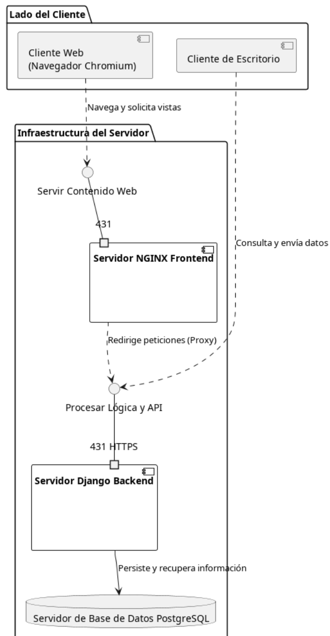
Figura 24: Diagrama de componentes y conectores.
