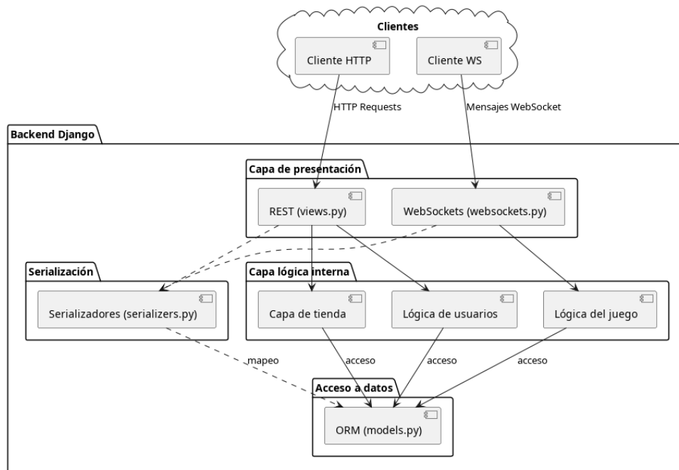
Figura 26: Diagrama de módulos del Backend.
