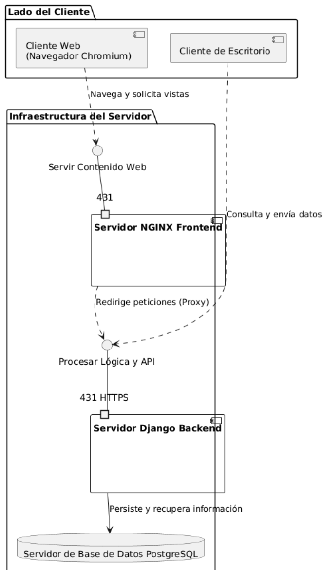
Figura 13: Diagrama de componentes y conectores.
