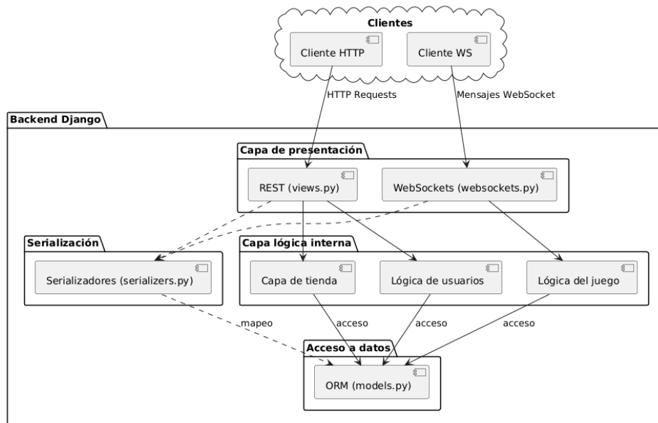
Figura 15: Diagrama de módulos del Backend.
