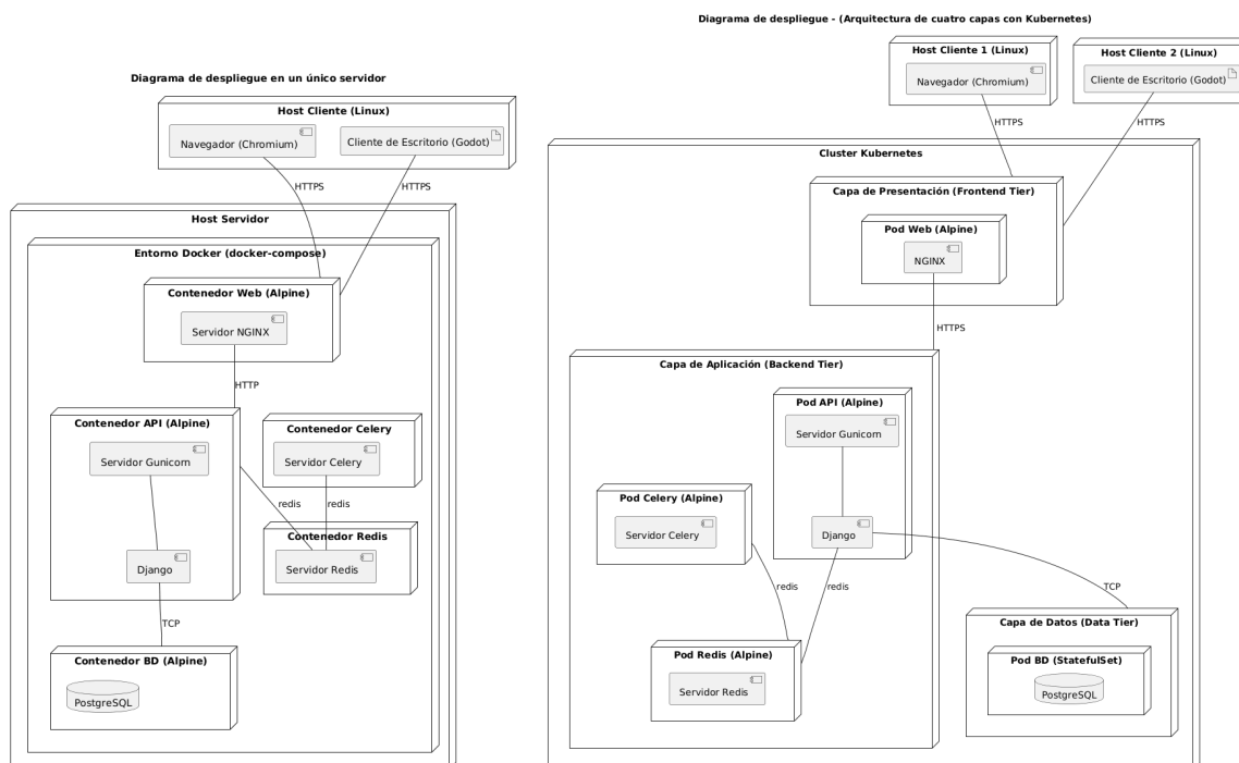
Figura 7: Diagramas de despliegue. A la izquierda, diagrama en 2 capas, como se realizará el despliegue, y a la derecha, en 4 capas, señalando las posibilidades de despliegue.
