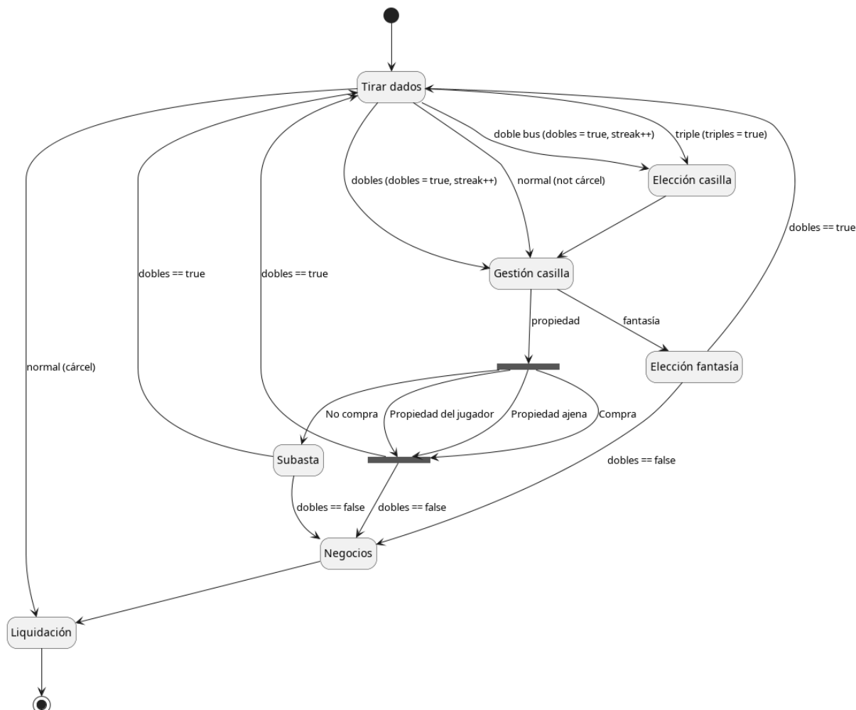
Figura 3: Diagrama de estados de un turno de juego con sus fases.
