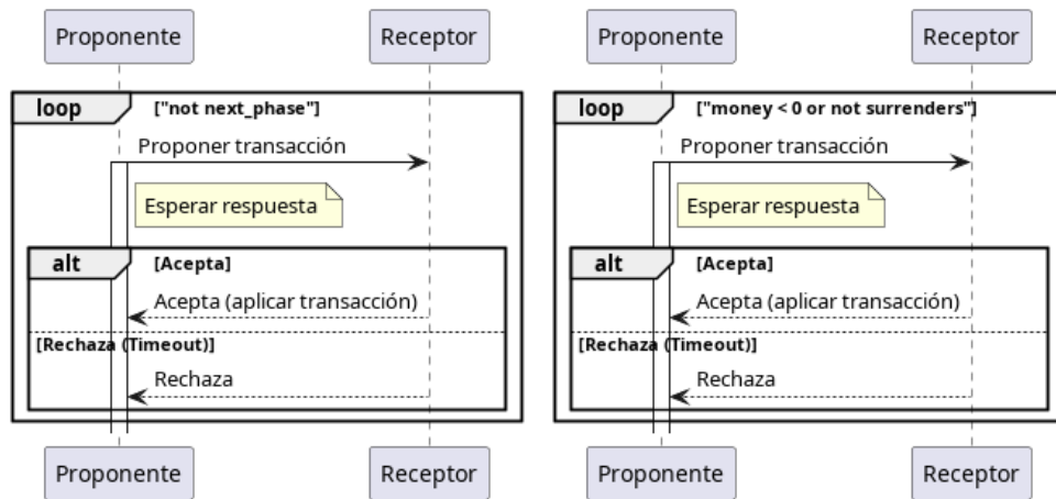
Figura 4: Diagramas de secuencia de las fases de negocios (izquierda) y liquidación (derecha).
