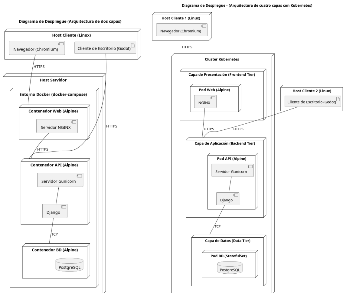
Figura 5: Diagramas de despliegue. A la izquierda, diagrama en 2 capas, como se realizará el despliegue, y a la derecha, en 4 capas, señalando las posibilidades de despliegue.
