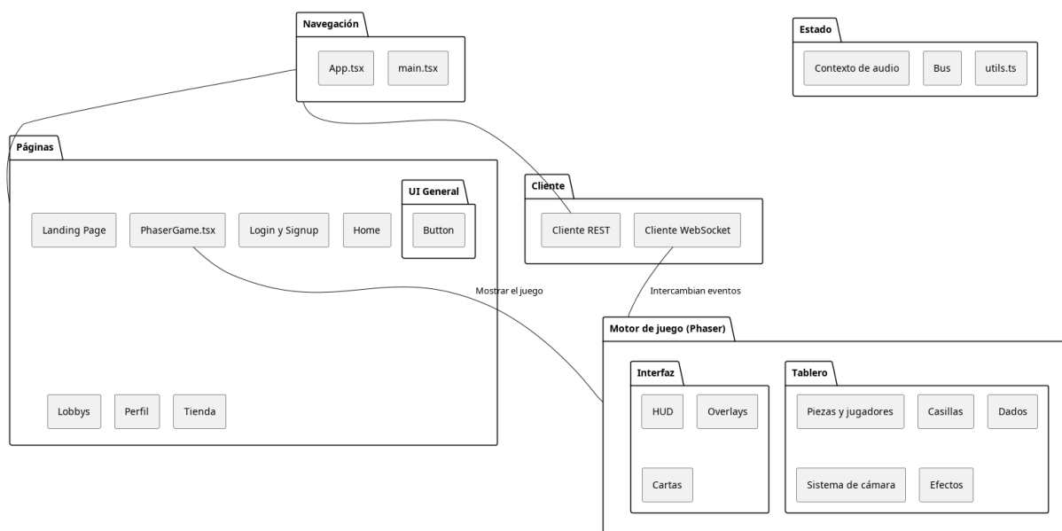
Figura 15: Diagrama de módulos del cliente web.
