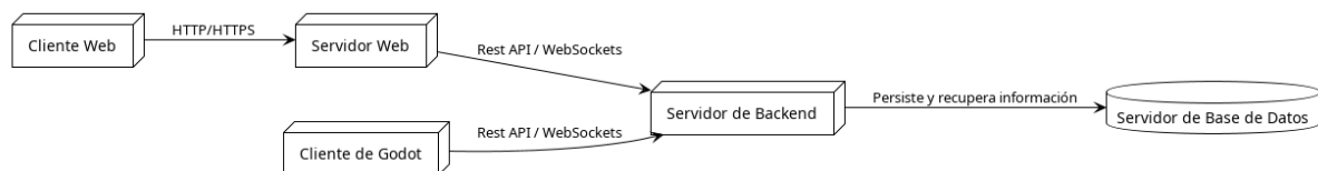
Figura 2: Diagrama de la arquitectura a alto nivel.
