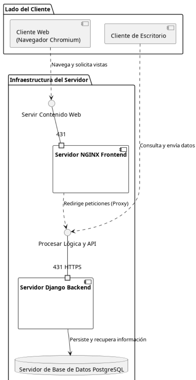
Figura 11: Diagrama de componentes y conectores.
