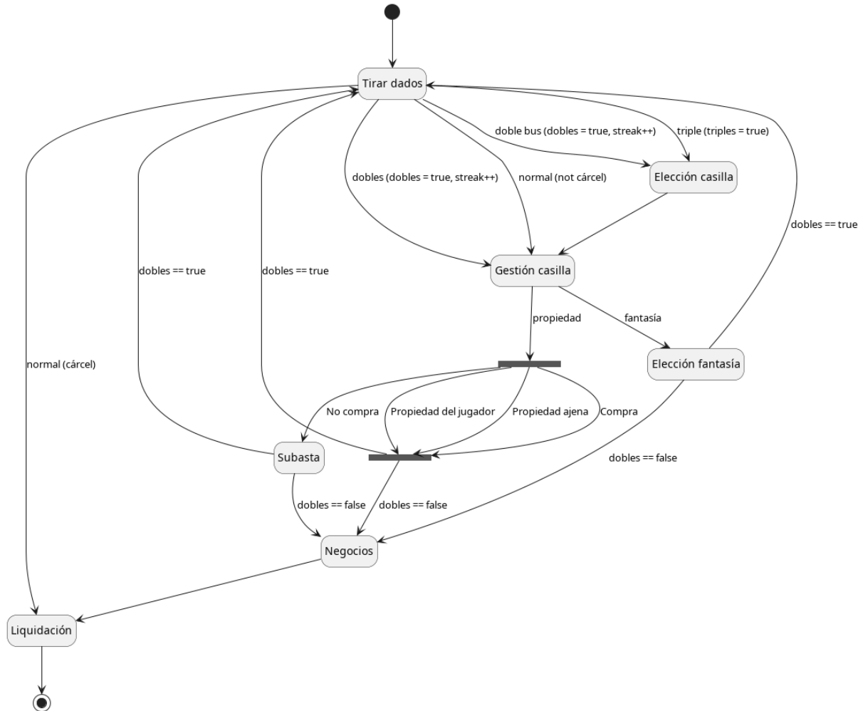
Figura 4: Diagrama de estados de un turno de juego con sus fases.
