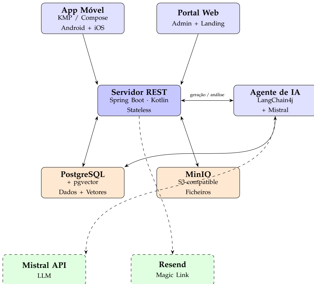
Figura 3.2: Arquitetura do Play4Change (C4 — Nível Contentor)
