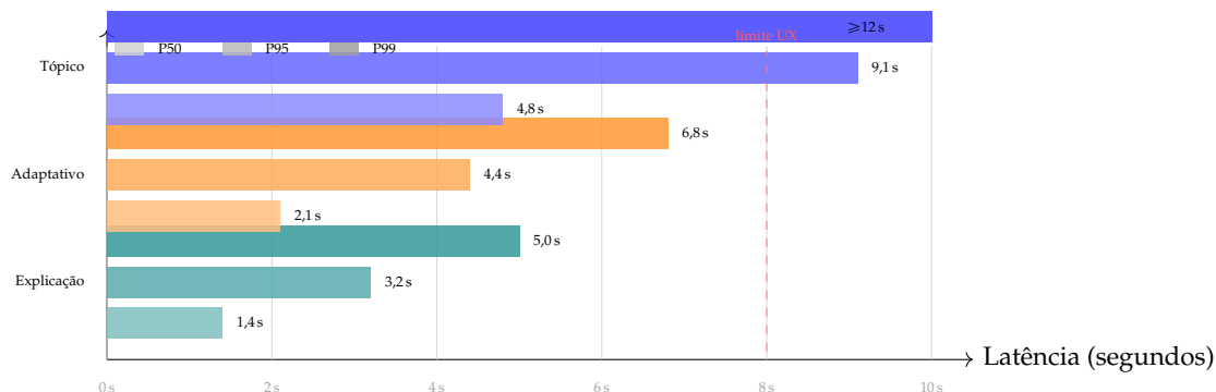
Figura 3.9: Percentis de latência de inferência do mistral-small-latest observados durante o período de avaliação, por tipo de chamada. A linha a tracejado assinala os 8 segundos como limiar prático de tolerância do utilizador para respostas interactivas [14]. Nota: os valores apresentados são representativos do período de avaliação; substituir pelos dados exactos exportados do Grafana/Prometheus antes de submeter o relatório final.
