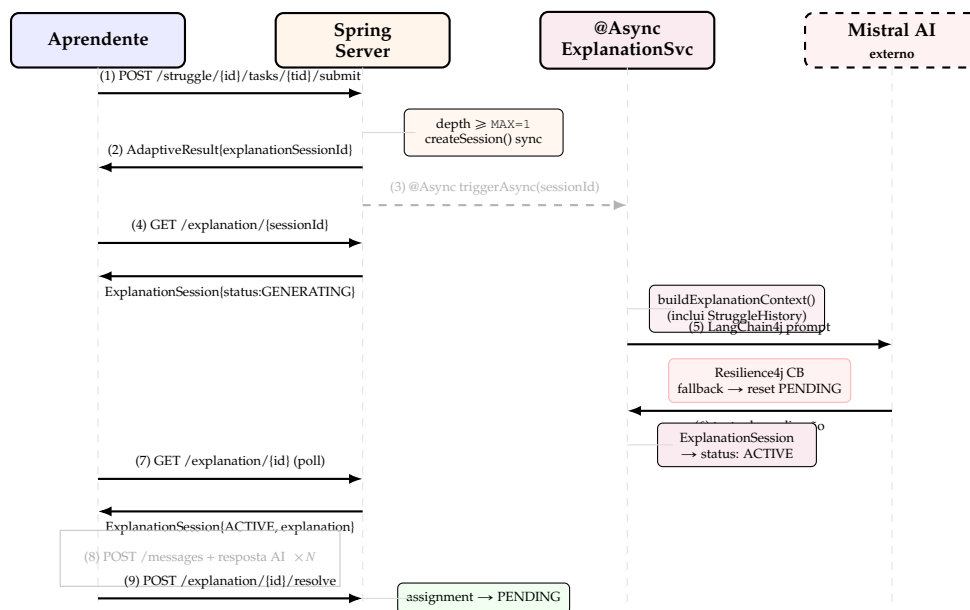
Figura 3.14: Diagrama de sequência da sessão de explicação. A criação da sessão é síncrona (passo 2), permitindo navegação imediata no cliente; a geração do texto holístico é assíncrona (@Async, passos 3–6), com fallback automático em caso de falha. Após transição para ACTIVE , decorre um número N de rondas de diálogo com o LLM (passo 8); a resolução (passo 9) repõe a tarefa original em PENDING para nova tentativa autónoma.
