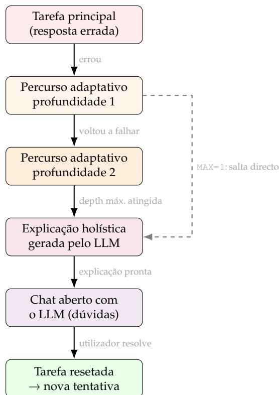
Figura 3.13: Escalada progressiva do percurso adaptativo para o modo de explicação: com \text{MAX\_STRUGGLE\_DEPTH} = 1 , após uma única falha no percurso adaptativo, o sistema escala directamente para a sessão de explicação e o diálogo com o LLM.
