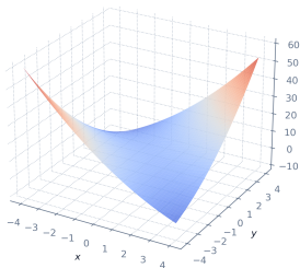
Superficie 3D (Punto de Silla)
