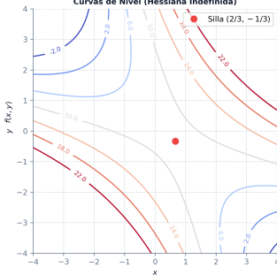
Curvas de Nivel (Hessiana Indefinida)
