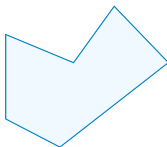
Conjunto NO Convexo \mathcal{S}
