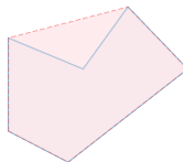
Envoltura Convexa \mathcal{H}(\mathcal{S})
