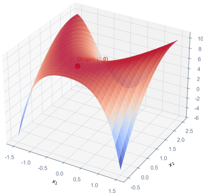
Función No Convexa en 3D f(x_1, x_2) = 10 - 2(x_2 - x_1^2)^2
