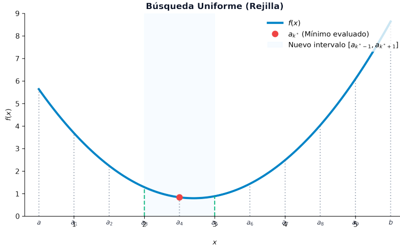
Figura 2.3: Concepto de la Búsqueda Uniforme en rejilla: subdivisión equidistante del intervalo y reducción basada en el punto mínimo de la muestra
