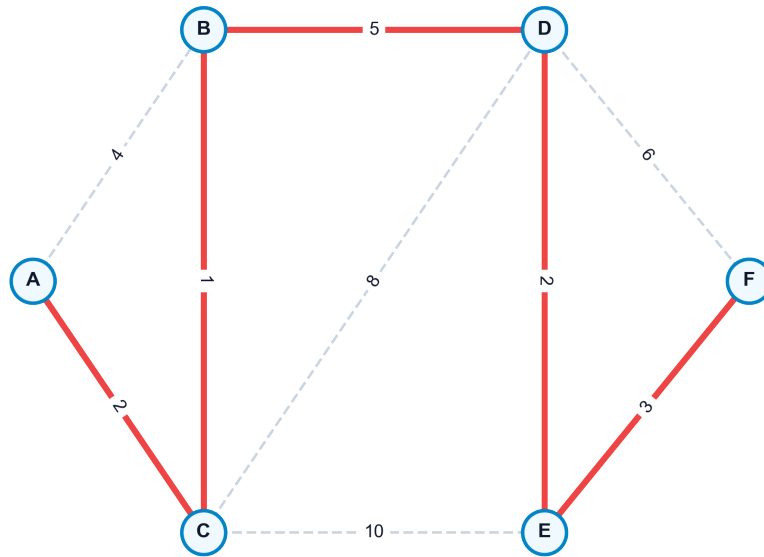
Figura 7.2: Árbol Soporte de Mínimo Peso (MST) destacado en color rojo sobre un grafo valorado
