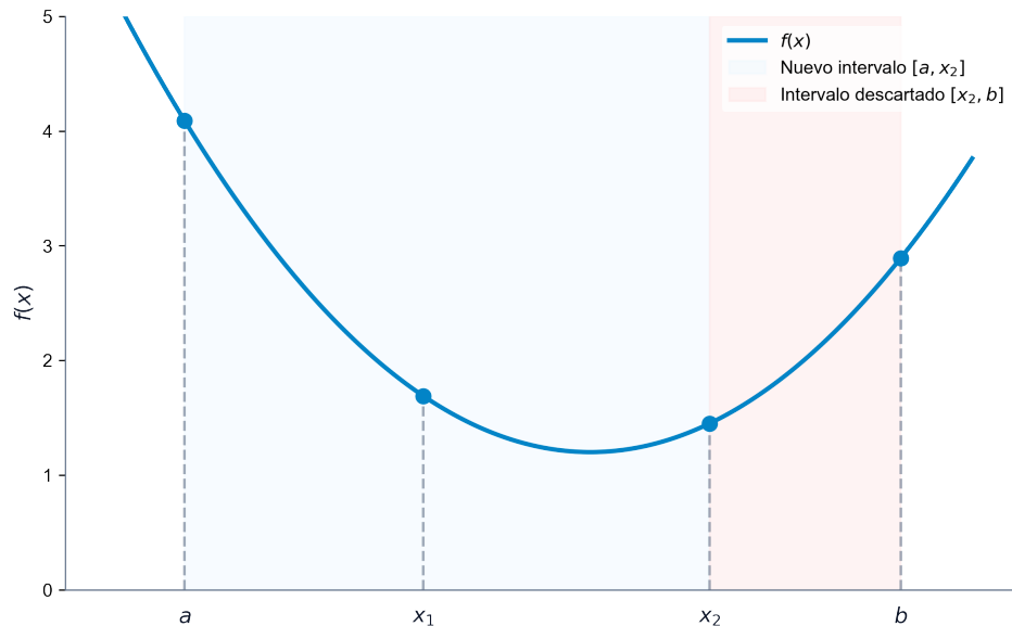
Figura 2.1: Búsqueda unidimensional y reducción de intervalos de incertidumbre
