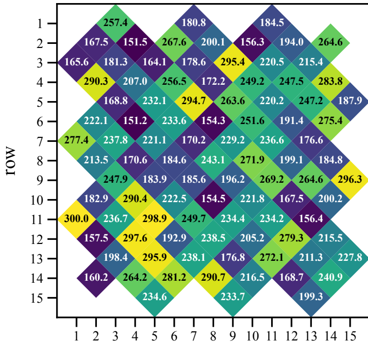
Qubit T_1 [us]
