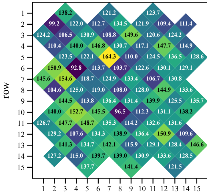
Qubit T_\phi [us]
