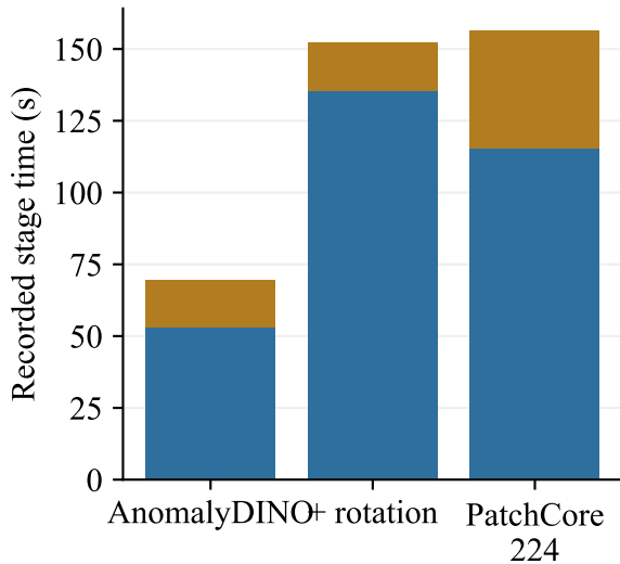
(b) BTAD
