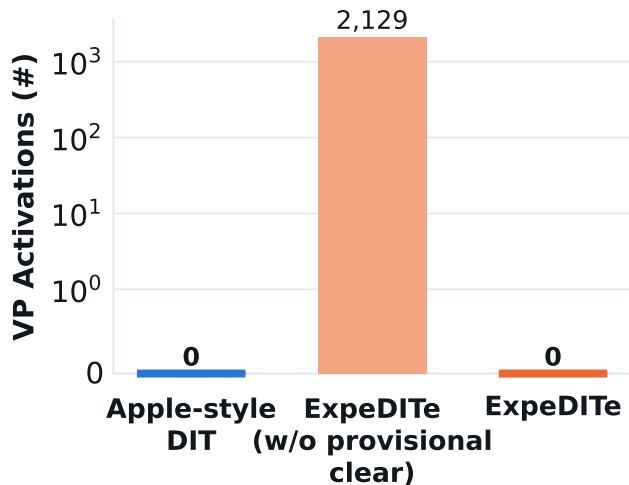
(d) Speculation on Clearing DIT
