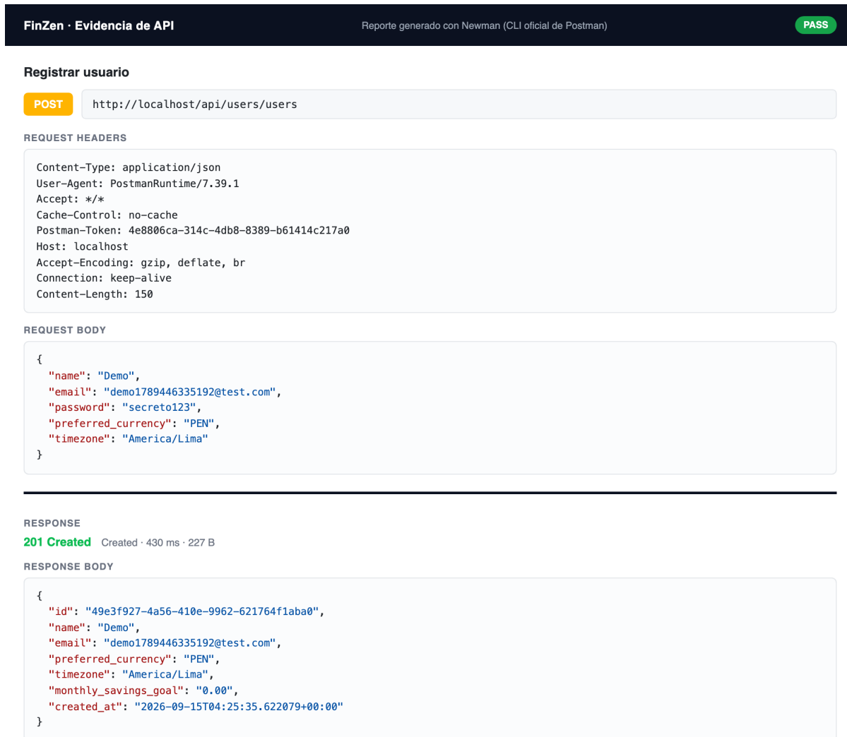
Figura 3: Registro de usuario (POST /api/users/users , 201 Created).
