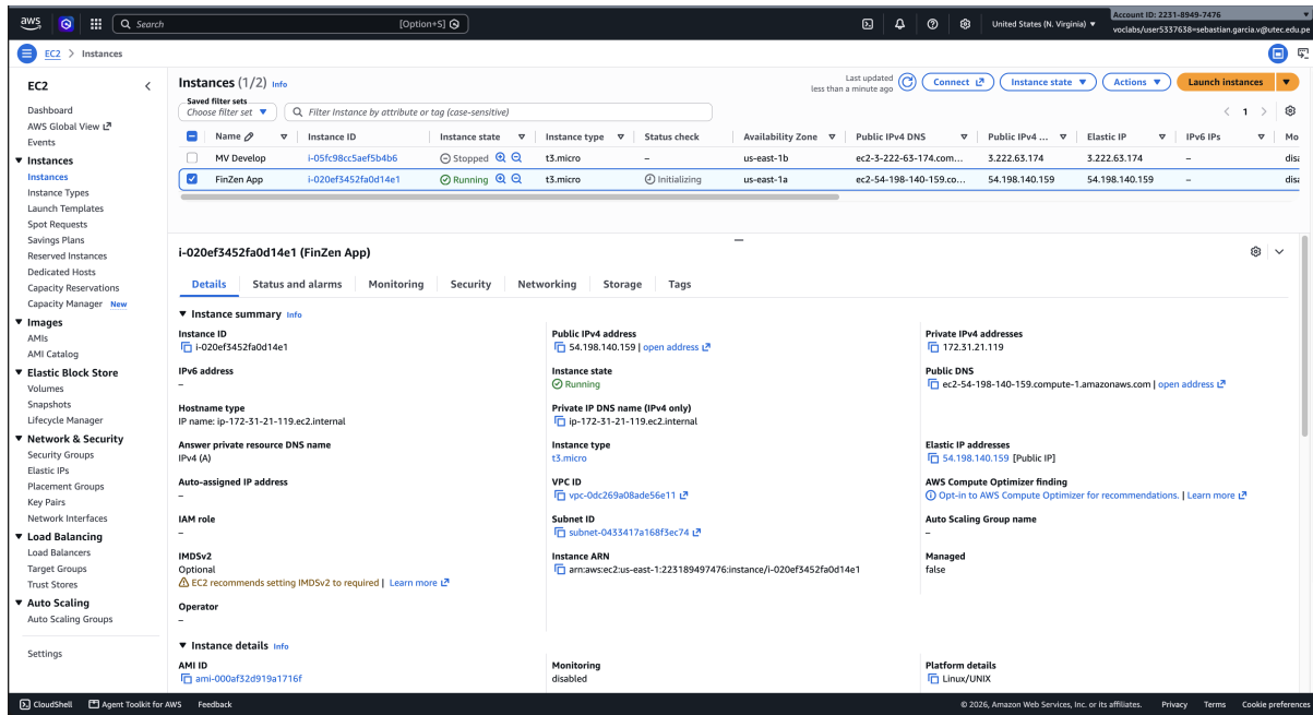
Figura 18: Consola de AWS (región us-east-1) con la instancia FinZen App en estado Running , tipo t3.micro y su IP elástica 54.198.140.159.
