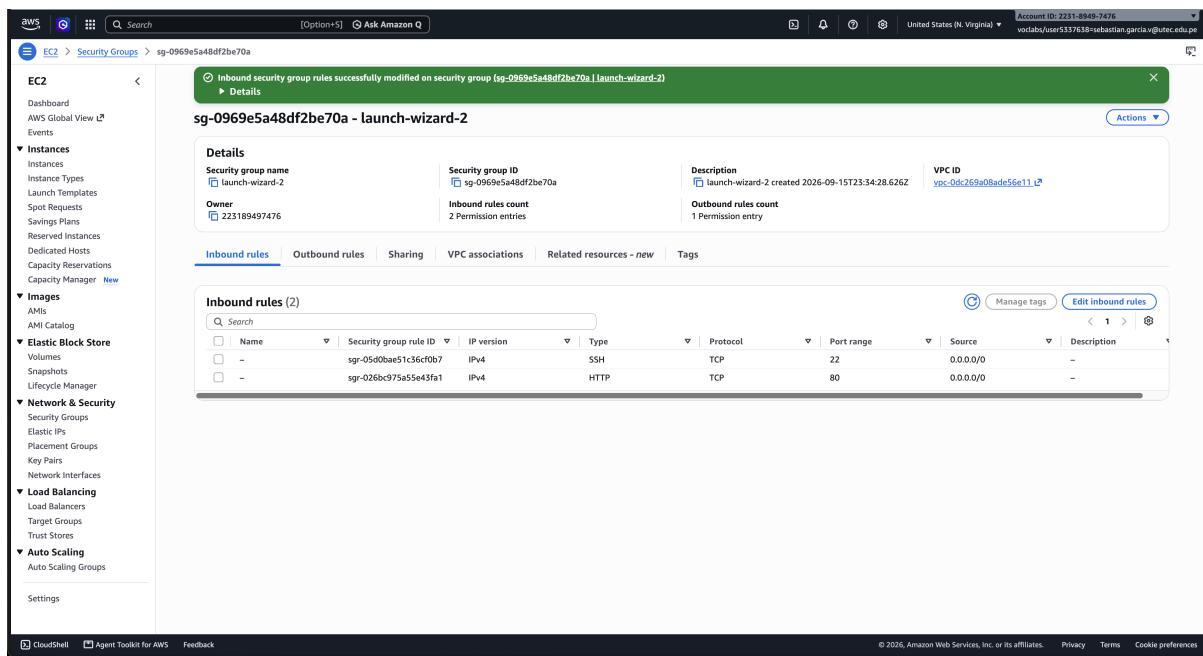
Figura 19: Reglas de entrada del Security Group: 22 (SSH) y 80 (HTTP), ambas desde 0.0.0.0/0.
