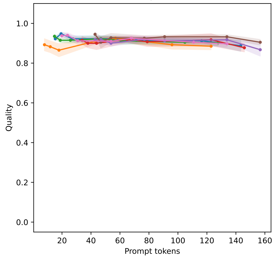
QA
