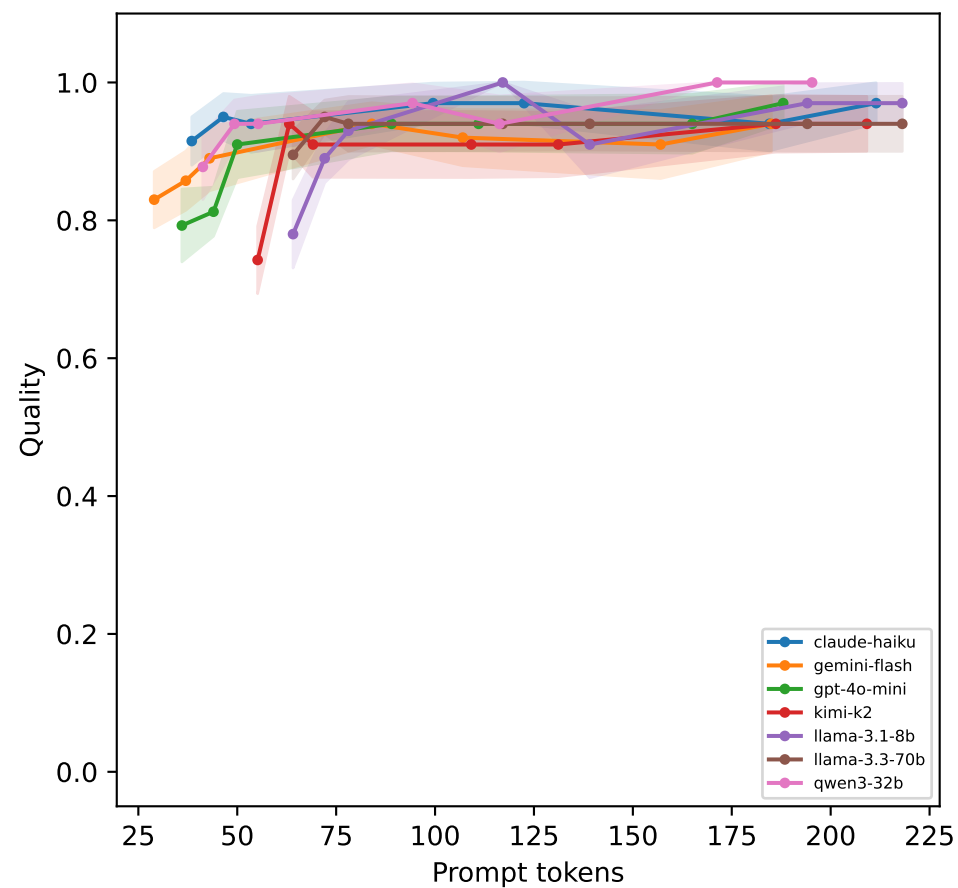
QA
