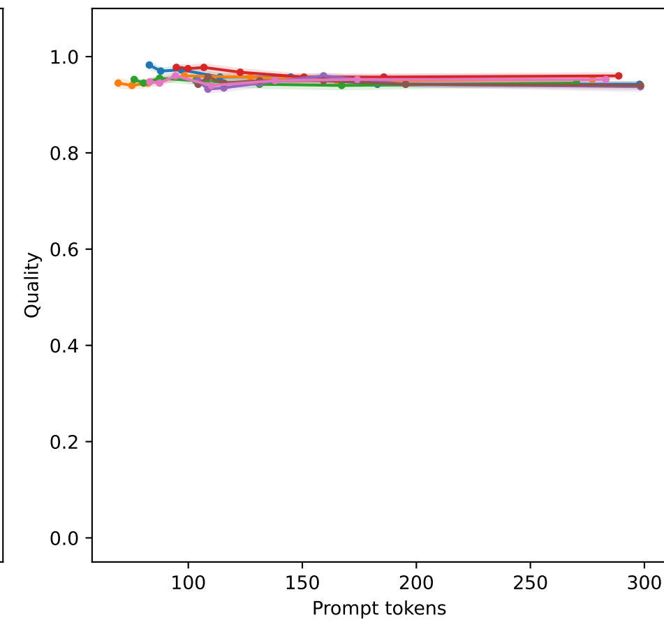
Summarisation
