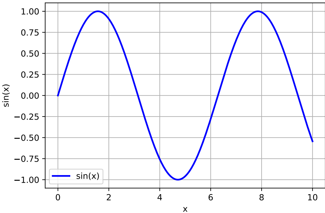
Funzione Sin(x)
